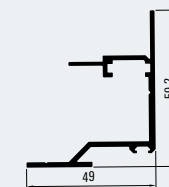
Rahmenprofil innen Frame profile inside 100023356
