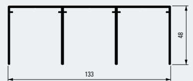
Führungsschiene 48, dreiläufig Guide track 48, triple track 100008395
