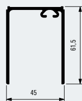
Führungsschiene 61, einläufig Guide track 61, single track 100022633
