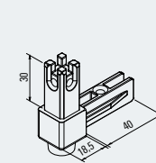
Eckknoten 2 S mit Stellfuß Corner joint, 2-sided with adjustable foot 100003075
