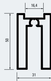
Rahmenprofil 16 unten für Rollenbeschlag Frame profile 16 bottom for roller fitting 100008685
