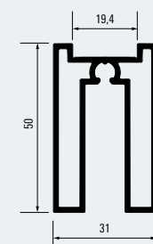
Rahmenprofil 19 unten für Rollenbeschlag Frame profile 19 bottom for roller fitting 100008720
