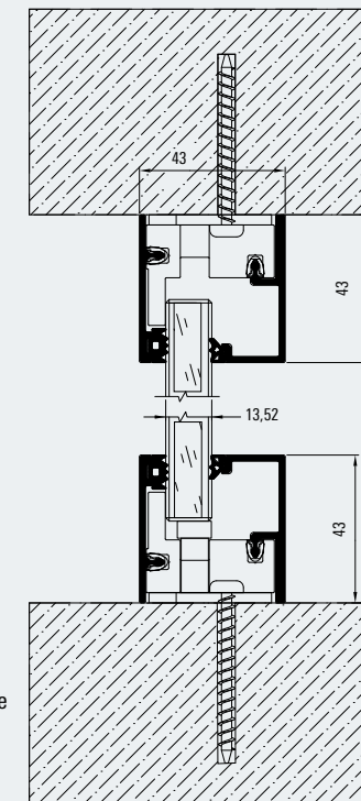
Glasschuh ohne Glasauflage Glass shoe without glass support 100023709 100023881
