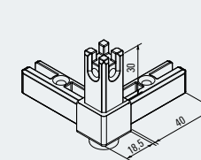
Eckknoten 3 S mit Stellfuß Corner joint, 3-sided with adjustable foot 100003069
