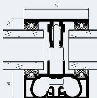
Horizontalschnitt Trägerprofil L Horizontal section detail of load-bearing profile L
