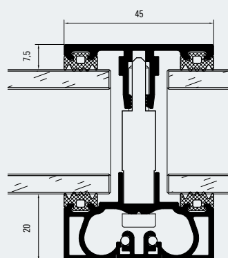
Horizontalschnitt Trägerprofil XL Horizontal section detail of load-bearing profile XL
