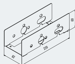
Schlosskasten für Türprofil Premium L-XL Lock case for premium door profile L-XL 100022604
