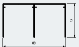
Führungsschiene 48, zweiläufig Guide track 48, double track 100008389
