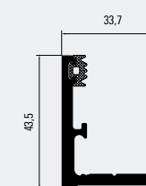
Grundprofil mit eingezogener Grunddichtung Basic profile with inserted basic gasket 100022301 mit/with 100021372
