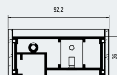
Horizontalschnitt unten Bottom horizontal section detail
