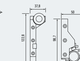
Slide Line M, Beschlagset ungedämpft Slide Line M, fittings kit not dampened 100002692
