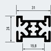
Sprossenprofil 19 Glazing bar profile 19 100008724
