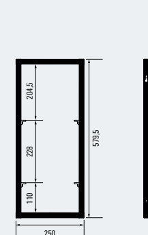
Set Seitenteil 580 mm Kit for 580 mm side section 100009235
