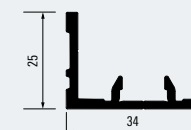
Aufsatzleiste Attachment rail 100008701
