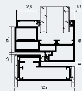
Horizontalschnitt oben Top horizontal section detail
