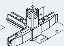
Eckknoten 4 S mit Stellfuß Corner joint, 4-sided with adjustable foot 100003072
