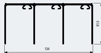
Führungsschiene 61, dreiläufig Guide track 61, triple track 100022573
