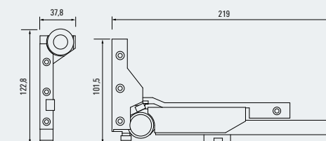
Slide Line M, Beschlagset gedämpft Slide Line M, fittings kit dampened 100002695
