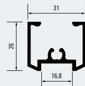
Rahmenprofil 16 oben / unten Frame profile 16 top / bottom 100008680
