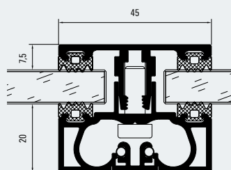
Horizontalschnitt Trägerprofil S Horizontal section detail of load-bearing profile S
