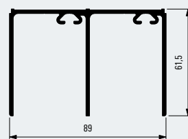
Führungsschiene 61, zweiläufig Guide track 61, double track 100008352
