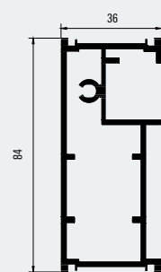
Türprofil unten Premium L-XL Premium bottom door profile L-XL 100022348
