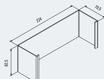
Abdeckung Schlosskasten für Türprofil Premium L-XL Cover for lock case for premium door profile L-XL 100022603
