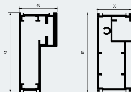
Türprofil Premium L-XL Premium door profile L-XL 100022346
