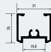
Rahmenprofil 19 oben / unten Frame profile 19 top / bottom 100008713
