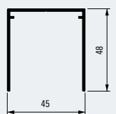
Führungsschiene 48, einläufig Guide track 48, single track 100008399
