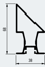
Griffprofil 45° Ecklösung auf Anfrage Handle profile 45° Corner solution on request 100023884
