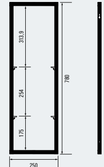
Set Seitenteil 780 mm Kit for 780 mm side section 100009607
