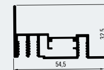
Rahmenprofil außen Frame profile outside 100023358
