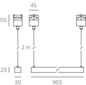
Adjustable cable. Cavo regolabile.
